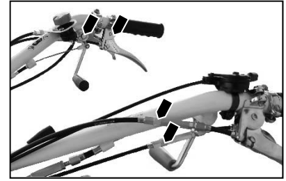
前輪上部ニップル、前単輪軸
