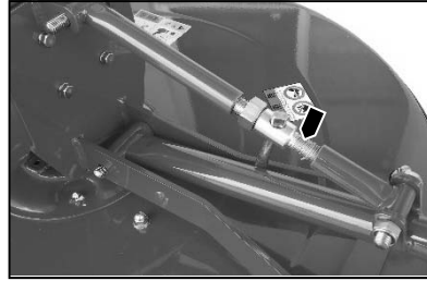
刈高調整ボルト
